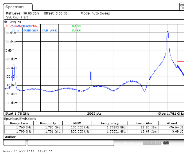
Band66-20MHz-QPSK-132572-1RB#99-PASS
