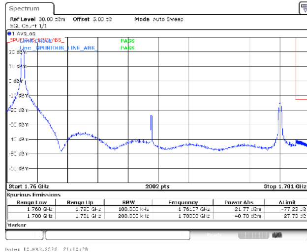
Band66-20MHz-QPSK-132572-1RB#0-PASS
