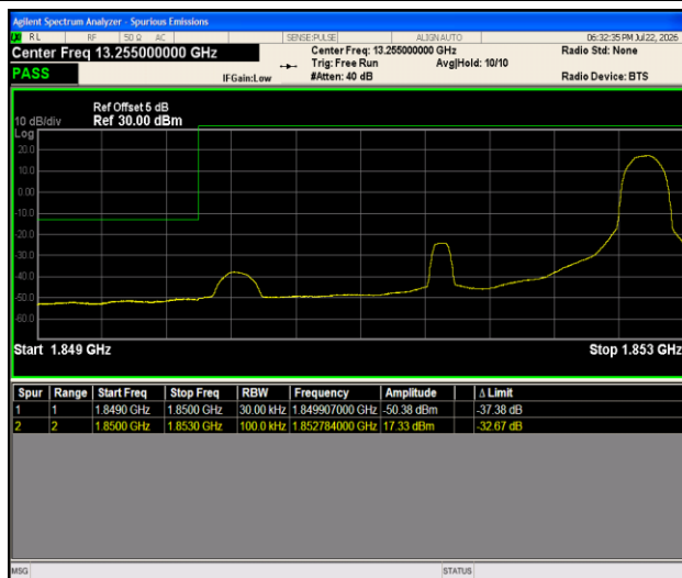
Band2-3MHz-16QAM-18615-1RB#14-PASS
