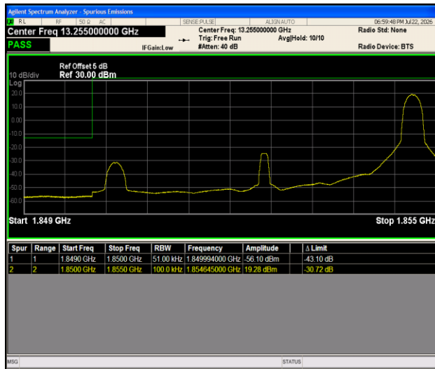
Band2-5MHz-QPSK-18625-1RB#24-PASS
