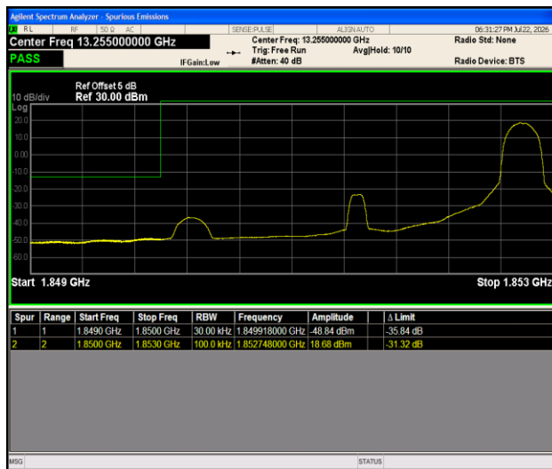
Band2-3MHz-QPSK-18615-1RB#14-PASS
