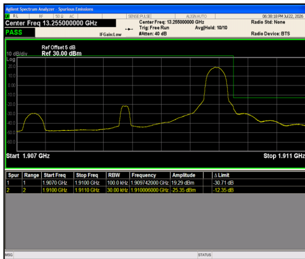
Band2-3MHz-QPSK-19185-1RB#14-PASS
