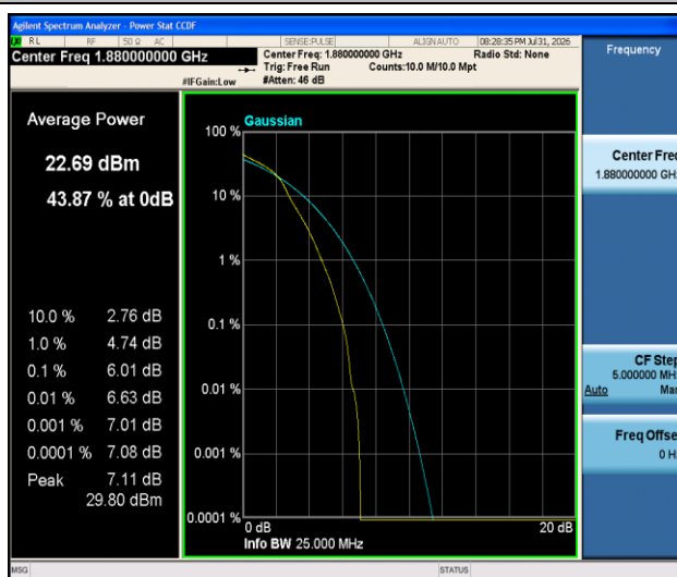
Band2-20MHz-16QAM-18900-1RB#0-PASS
