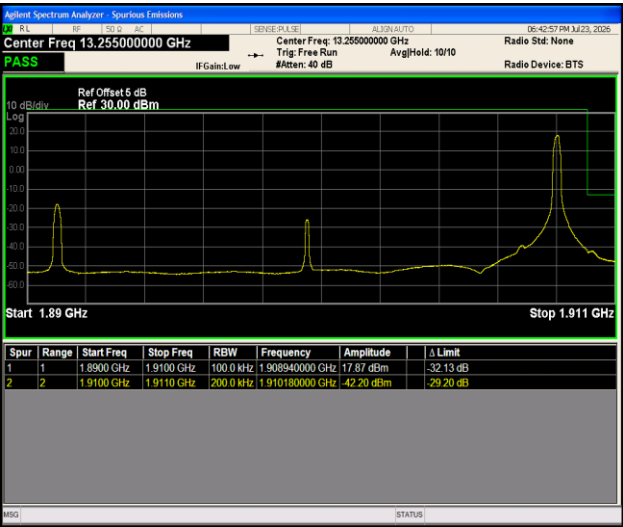
Band2-20MHz-16QAM-19100-1RB#99-PASS
