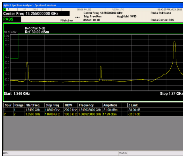
Band2-20MHz-16QAM-18700-1RB#99-PASS
