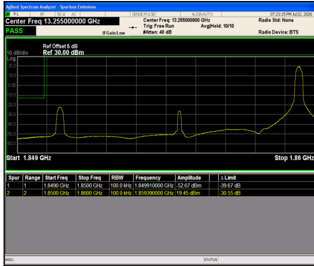
Band2-10MHz-QPSK-18650-1RB#49-PASS
