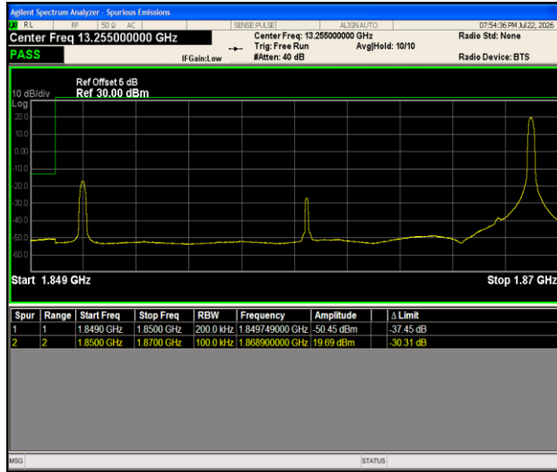
Band2-20MHz-QPSK-18700-1RB#99-PASS
