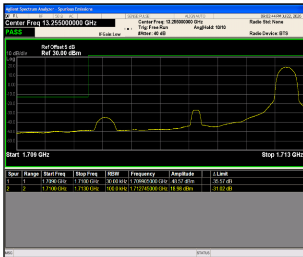
Band4-3MHz-QPSK-19965-1RB#14-PASS
