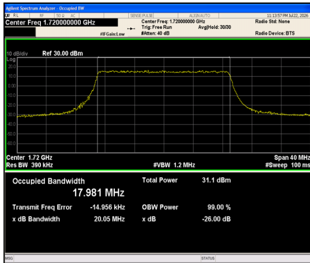
Band4-20MHz-QPSK-20050-100RB#0-PASS
