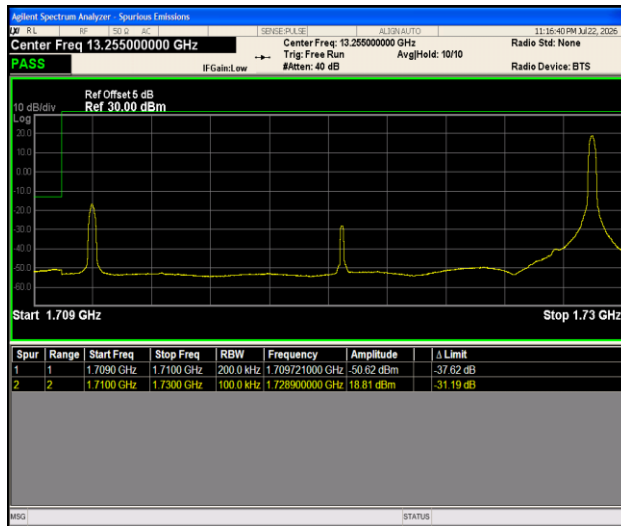
Band4-20MHz-QPSK-20050-1RB#99-PASS
