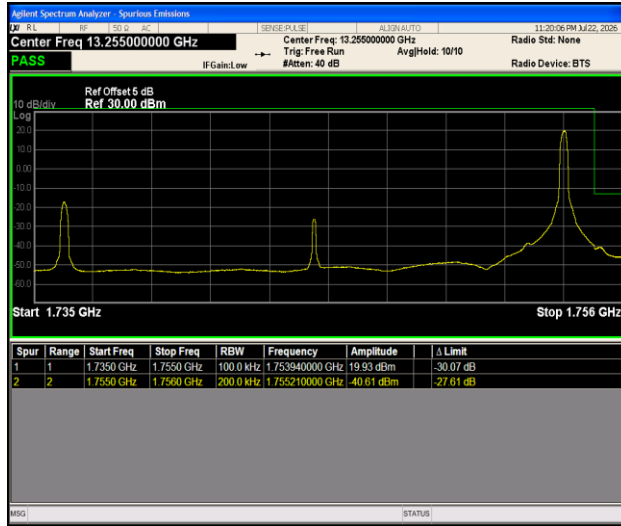
Band4-20MHz-QPSK-20300-1RB#99-PASS
