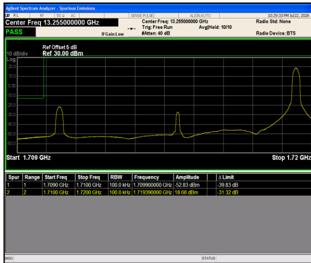
Band4-10MHz-QPSK-20000-1RB#49-PASS
