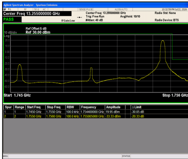
Band4-10MHz-QPSK-20350-1RB#49-PASS
