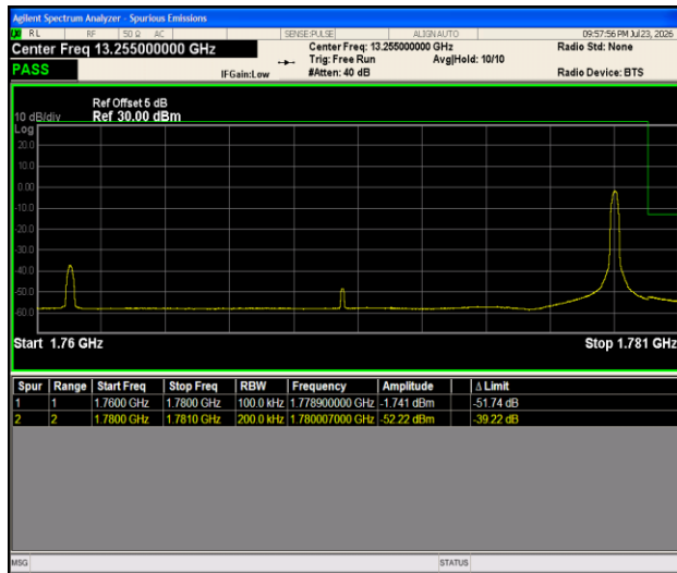
Band66-20MHz-QPSK-132572-1RB#99-PASS
