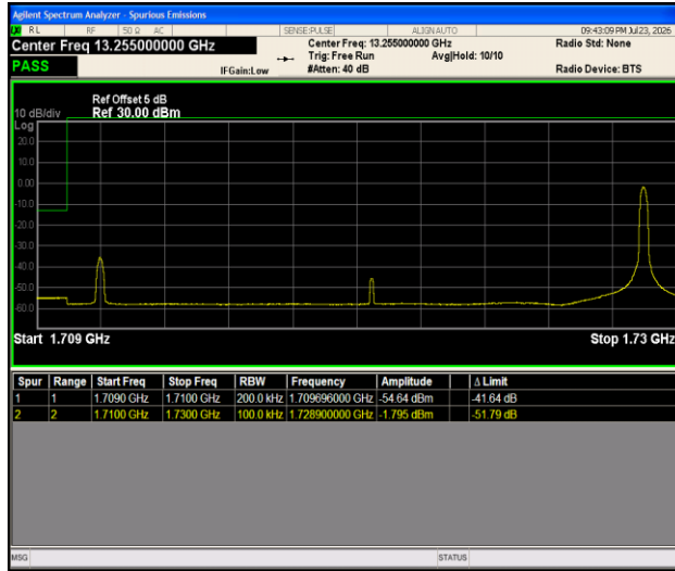
Band66-20MHz-QPSK-132072-1RB#99-PASS
