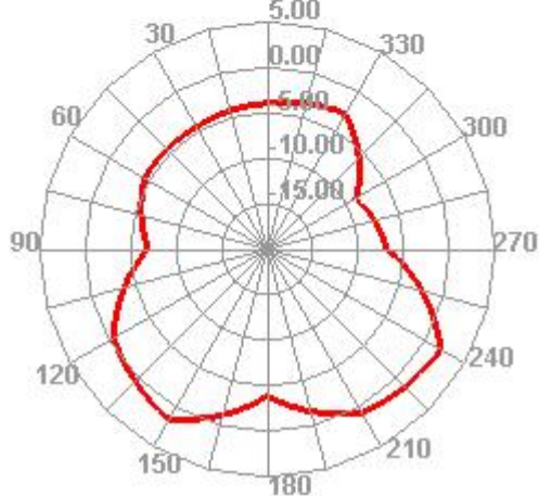
2400.000MHz E2
