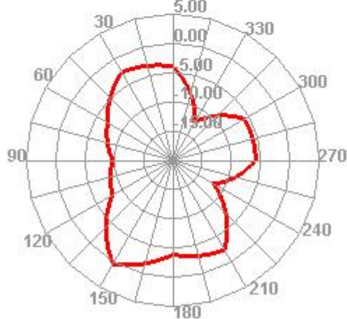
2400.000MHz E1
