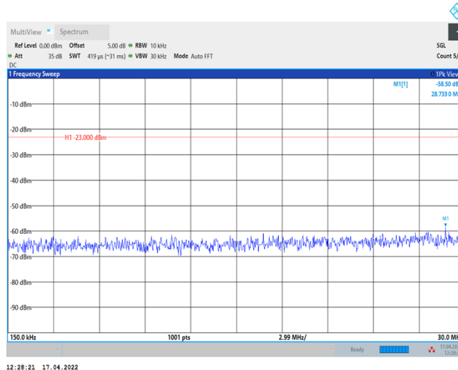
Band25-20MHz-QPSK-26140-1RB#0-Range2:0.15~30MHz
