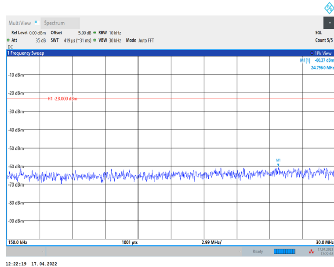
Band2-20MHz-QPSK-18700-1RB#0-Range2:0.15~30MHz
