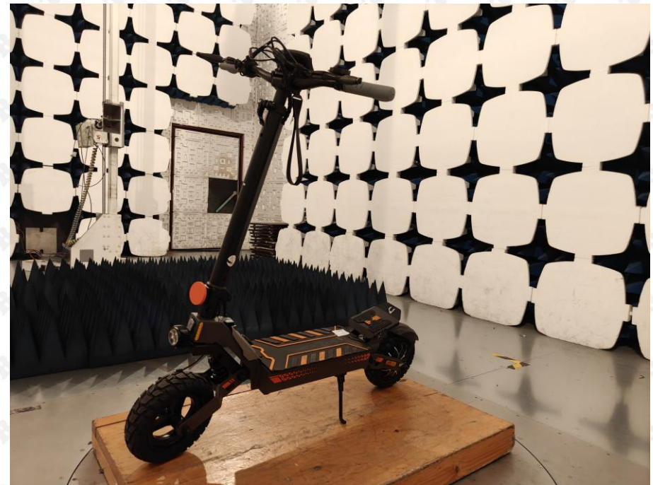
Above 1G
