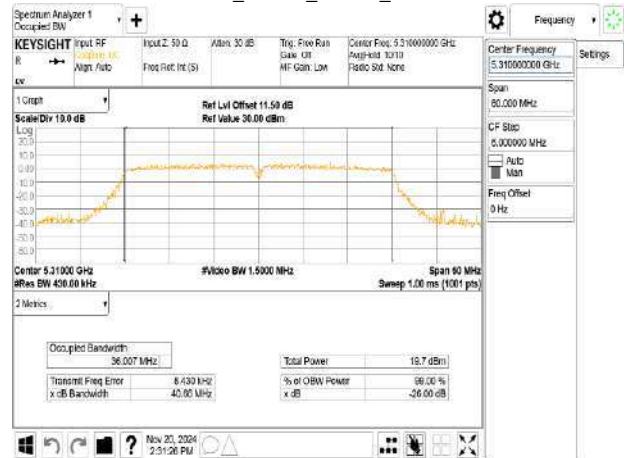
802.11n_40MHz_Chain1_5310MHz
