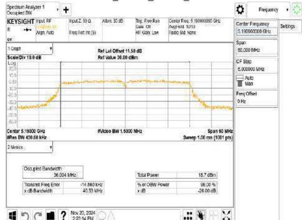
802.11n_40MHz_Chain1_5190MHz
