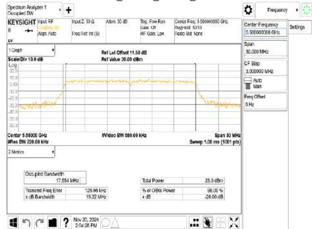
802.11n_20MHz_Chain1_5580MHz
