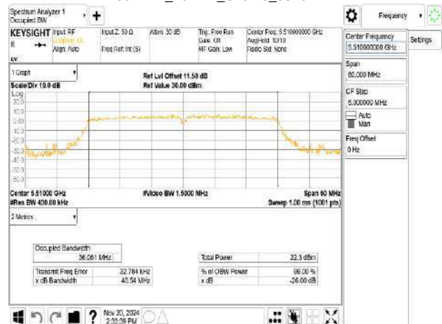
802.11n_40MHz_Chain0_5510MHz
