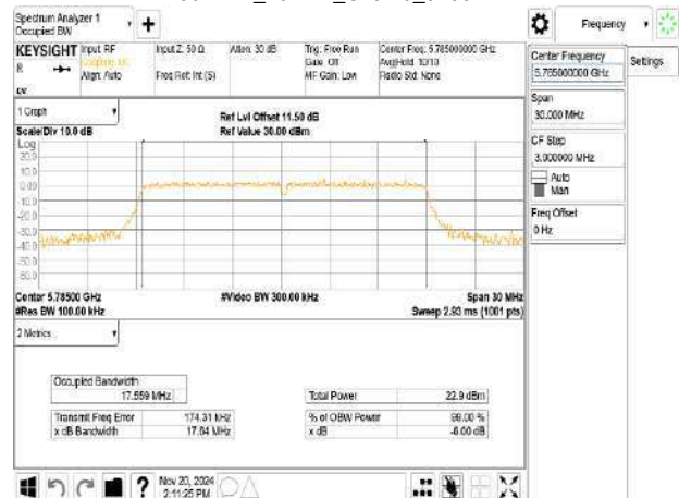
802.11n_20MHz_Chain0_5785MHz
