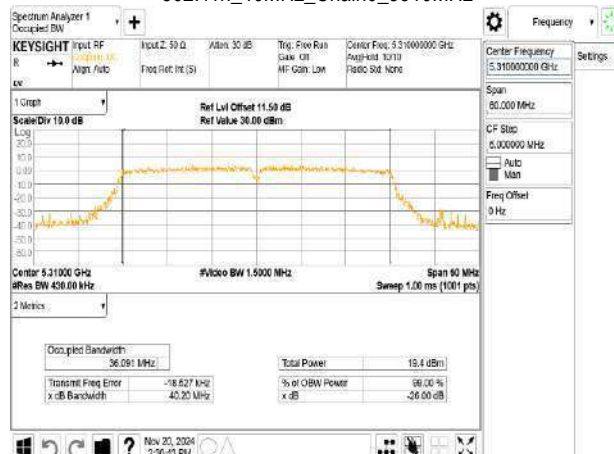
802.11n_40MHz_Chain1_5310MHz
