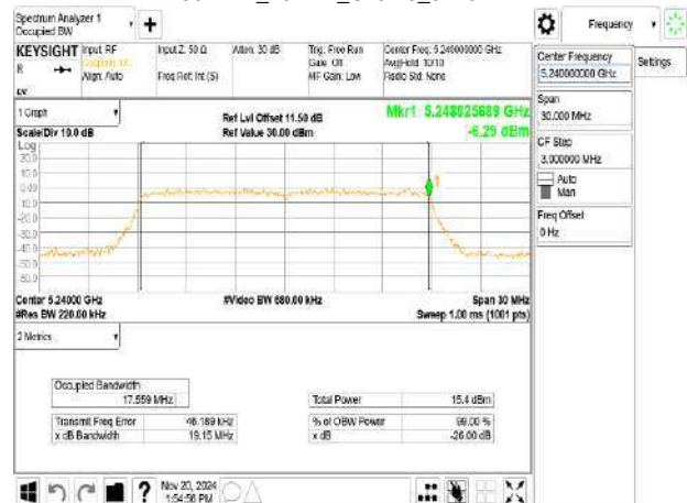
802.11n_20MHz_Chain0_5240MHz
