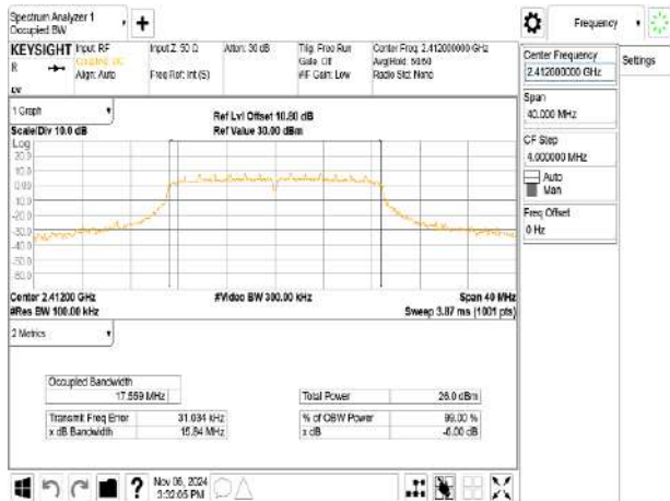
802.11n_20MHz_Chain1_2412MHz
