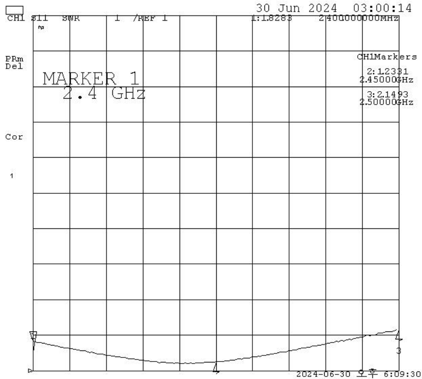
VSWR
