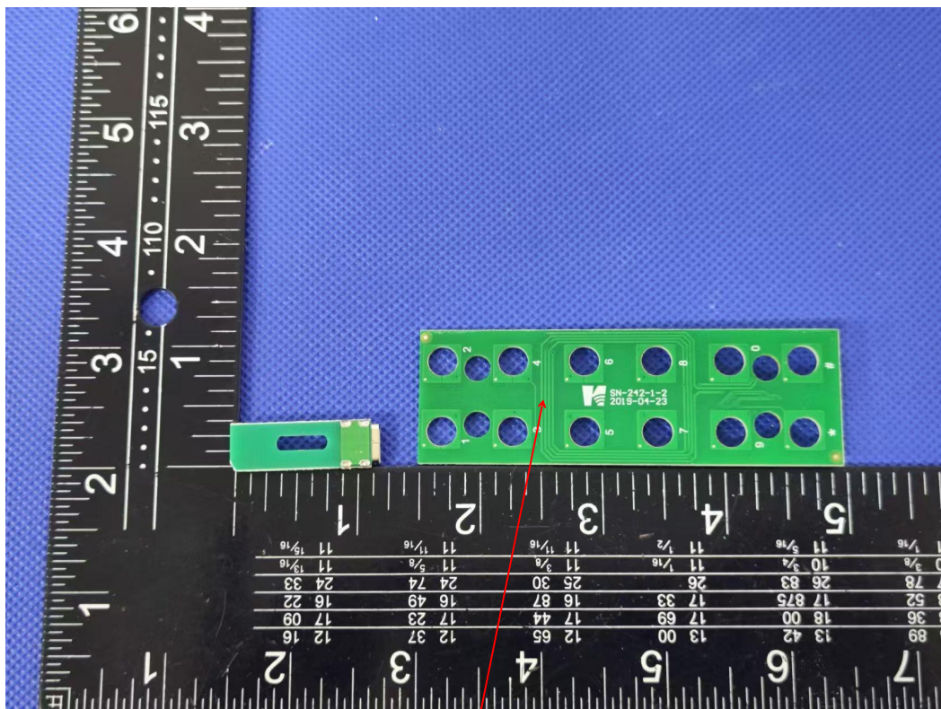
NFC Antenna
