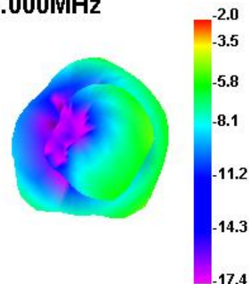
2400.000MHz H
