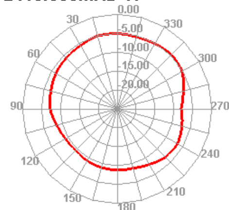
2410.000MHz H
