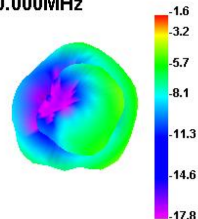
2410.000MHz H
