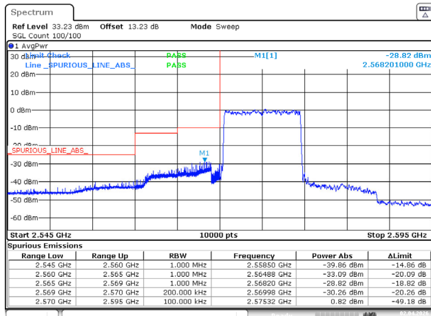
10MHz_Low_QPSK_50@0
