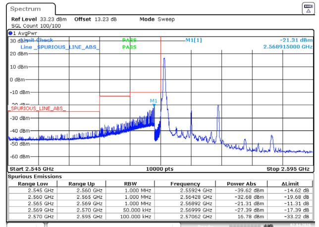
10MHz_Low_QPSK_1@0
