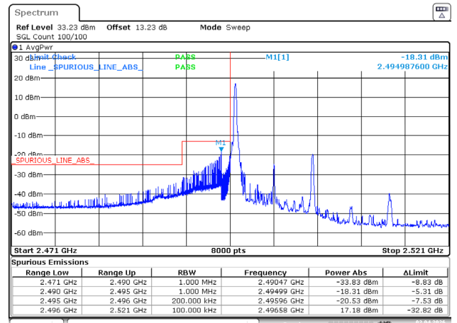
10MHz_Low_QPSK_1@0
