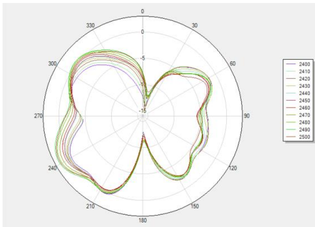
天线 2440MHz 2D-Phi Pattern
