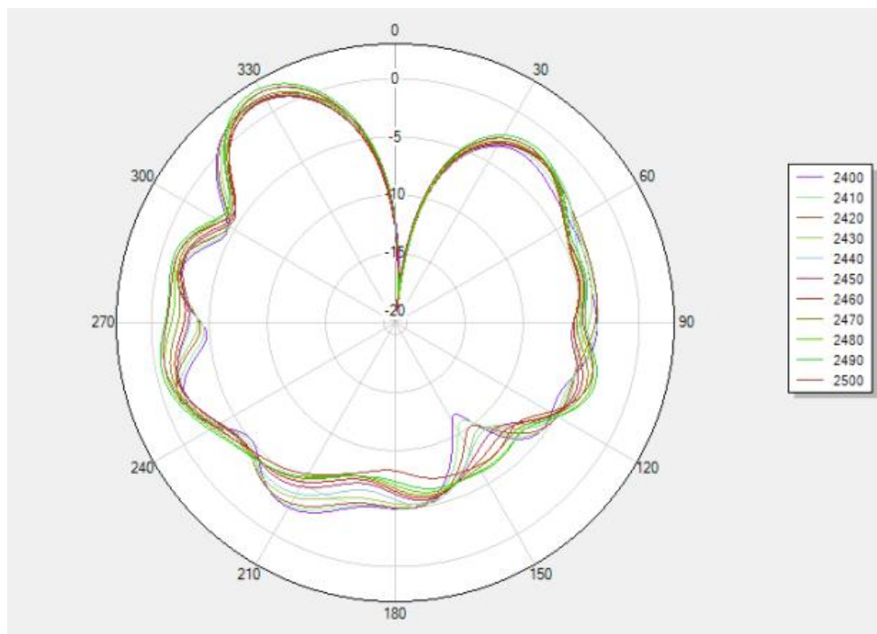
天线 2440MHz 2D-Theta Pattern
