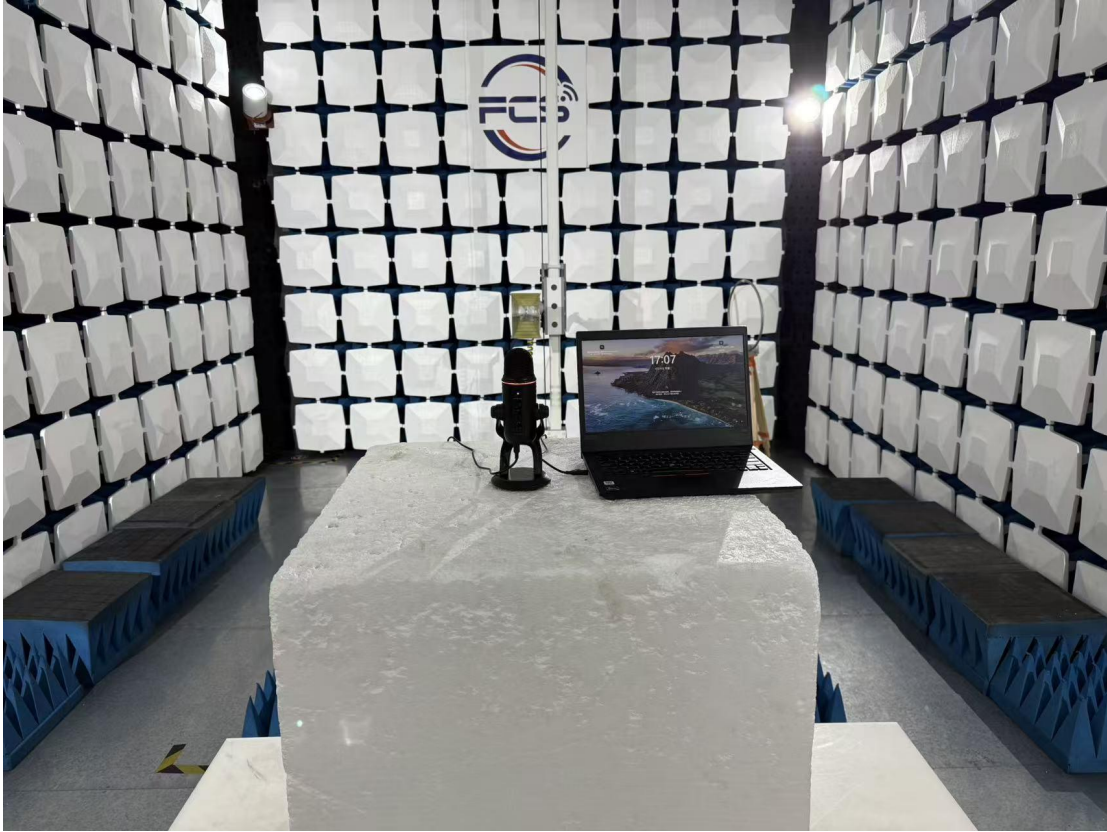
RE (Below1GHz)
