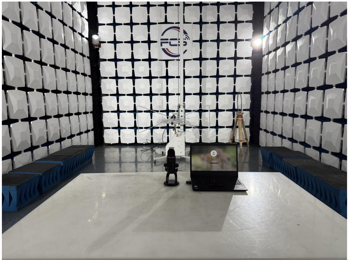
RE (Below1GHz)
