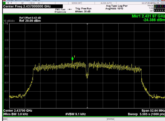
IEEE 802.11n_Channel 6_40MHz_Antenna 2
