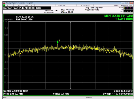
IEEE 802.11b_Channel 6_20MHz_Antenna 2
