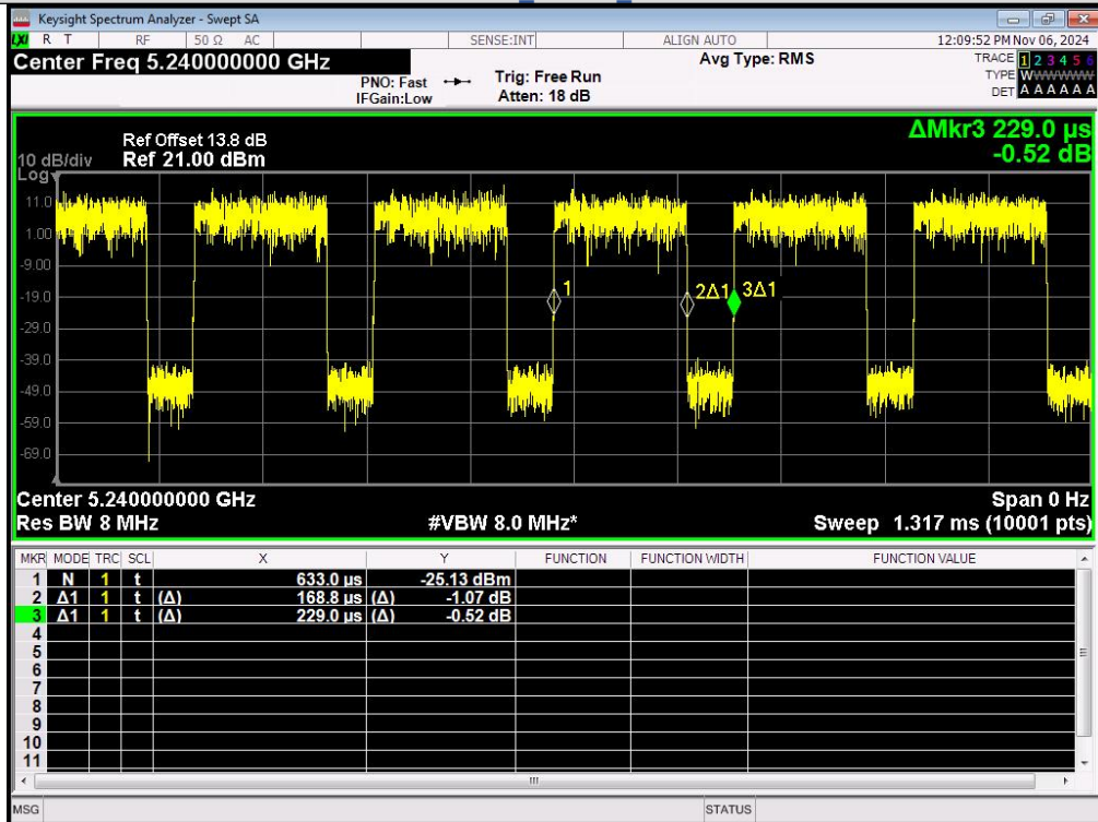
IEEE 802.11ac_20MHz_Channel 48
