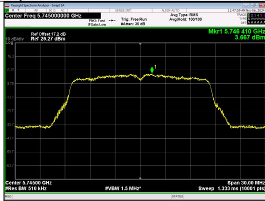
IEEE 802.11a Channel 149 20MHz Antenna 3
