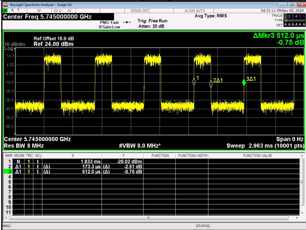
IEEE 802.11ac_20MHz_Channel 149
