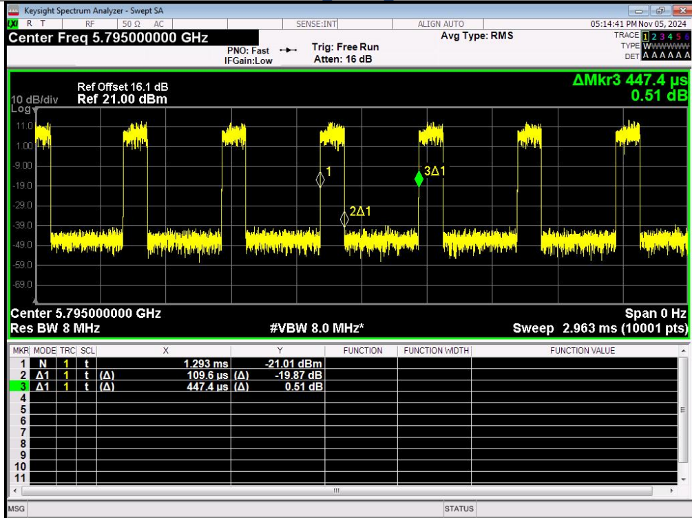
IEEE 802.11ac_40MHz_Channel 159
