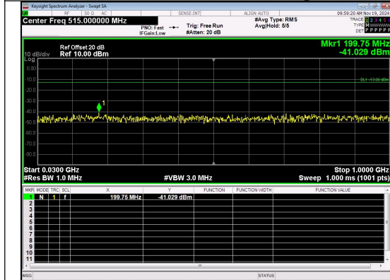
30.0MHz-1000.0MHz Band 4 20MHz/1745.0/1000.0MHz High QPSK 1@0
