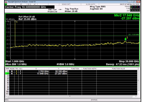
1000.0MHz-20000.0MHz Band 4 15MHz/1717.5/20000.0MHz Low 16QAM 1@0
