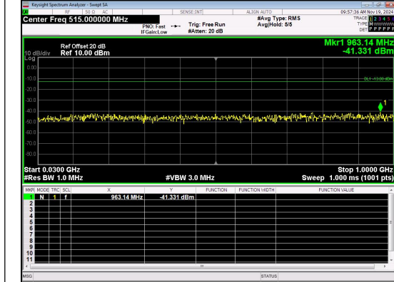
30.0MHz-1000.0MHz Band 4 15MHz/1717.5/1000.0MHz Low 16QAM 1@0
