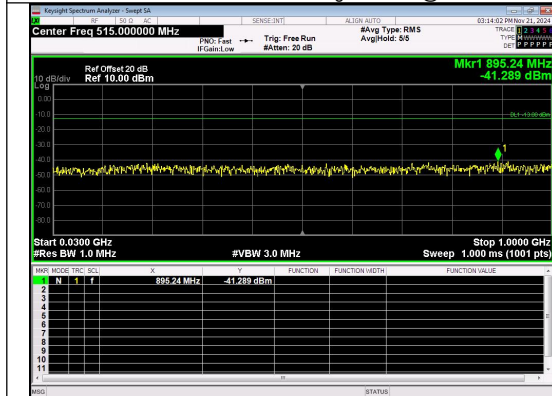
30.0MHz-1000.0MHz Band 4 20MHz/1745.0/1000.0MHz High 16QAM 1@0
