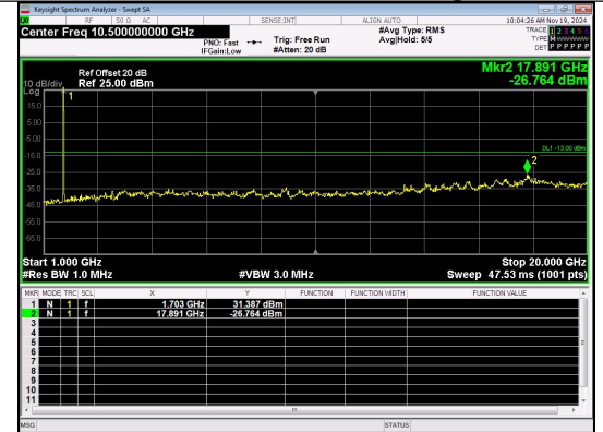
1000.0MHz-20000.0MHz Band 4 20MHz/1732.5/Mid 16QAM 1@0
