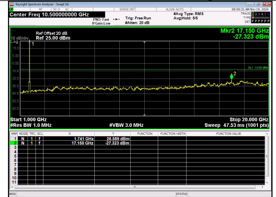
1000.0MHz-20000.0MHz Band 4 20MHz/1745.0/20000.0MHz High QPSK 1@0
