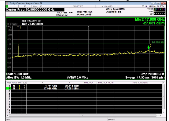
1000.0MHz-20000.0MHz Band 4 20MHz/1745.0/20000.0MHz High 16QAM 1@0
