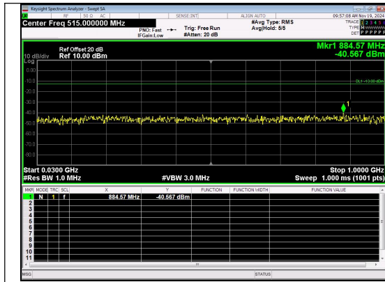
30.0MHz-1000.0MHz Band 4 15MHz/1717.5/1000.0MHz Low QPSK 1@0
