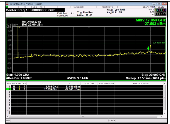
1000.0MHz-20000.0MHz Band 4 15MHz/1717.5/20000.0MHz Low QPSK 1@0
