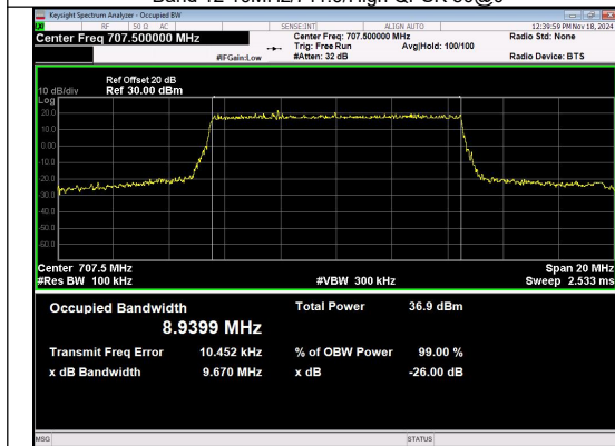
Band 12 10MHz/707.5/Mid QPSK 50@0
