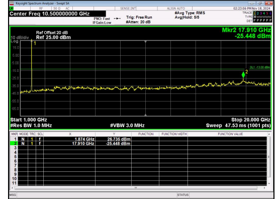
1000.0MHz-20000.0MHz Band 2 10MHz/1880.0/Mid QPSK 1@0
