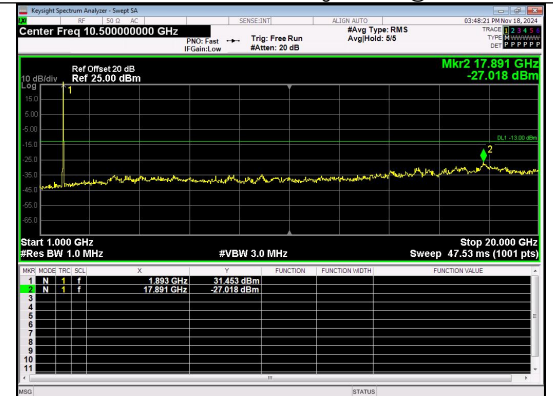
1000.0MHz-20000.0MHz Band 2 20MHz/1900.0/High 16QAM 1@0
