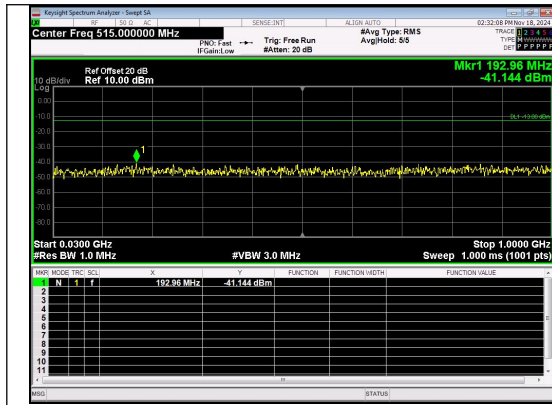
30.0MHz-1000.0MHz Band 2 15MHz/1857.5/Low QPSK 1@0
