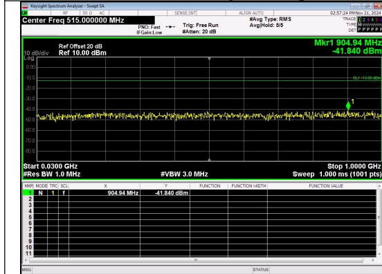
30.0MHz-1000.0MHz Band 2 15MHz/1880.0/Mid QPSK 1@0
