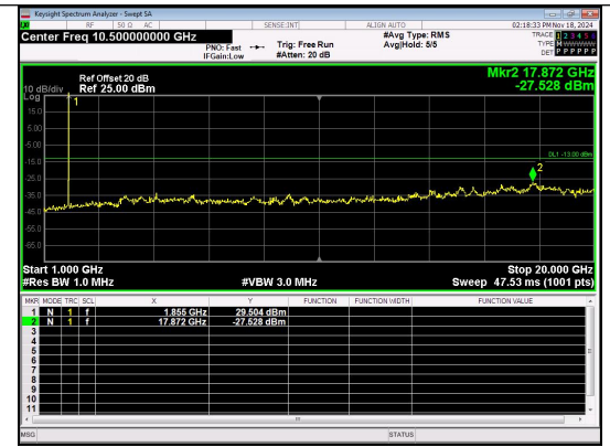
1000.0MHz-20000.0MHz Band 2 5MHz/1852.5/Low QPSK 1@0
