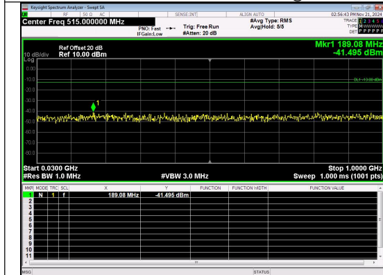
30.0MHz-1000.0MHz Band 2 10MHz/1855.0/Low QPSK 1@0
