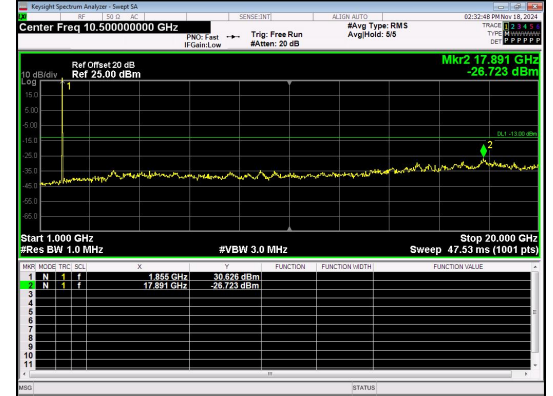
1000.0MHz-20000.0MHz Band 2 15MHz/1857.5/Low 16QAM 1@0
