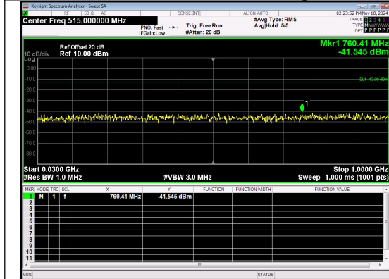
30.0MHz-1000.0MHz Band 2 10MHz/1880.0/Mid 16QAM 1@0
