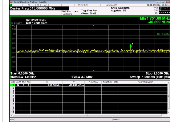
30.0MHz-1000.0MHz Band 2 10MHz/1880.0/Mid QPSK 1@0
