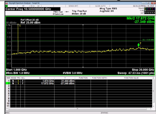
1000.0MHz-20000.0MHz Band 2 15MHz/1880.0/Mid 16QAM 1@0
