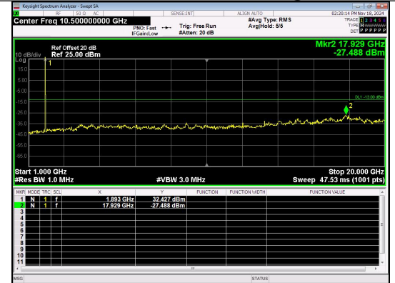
1000.0MHz-20000.0MHz Band 2 10MHz/1905.0/High QPSK 1@0
