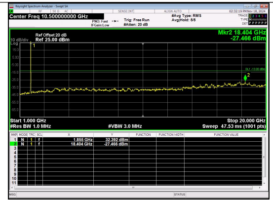
1000.0MHz-20000.0MHz Band 2 15MHz/1857.5/Low QPSK 1@0
