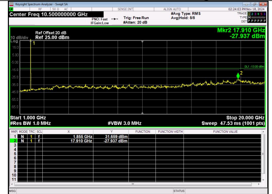
1000.0MHz-20000.0MHz Band 2 10MHz/1880.0/Mid 16QAM 1@0
