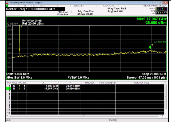
1000.0MHz-20000.0MHz Band 2 20MHz/1900.0/High QPSK 1@0
