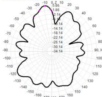
5850.0MHz Total(E1-XZ), Max= 5.86dBi
