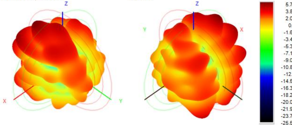
5850.0MHz Total(E1-XZ), Max= 3.29dBi
