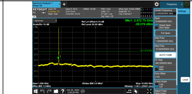
Band41(2555-2655)-10MHz-QPSK-40690-50RB#0-20000-2700-0-PASS
