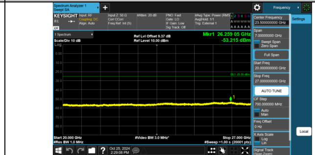
Band41(2555-2655)-10MHz-QPSK-40690-1RB#49-1000-10000-PASS
