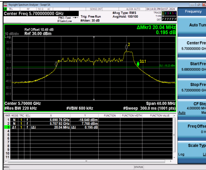
11AX20MIMO_Ant W0_5700_52Tone_RU40
