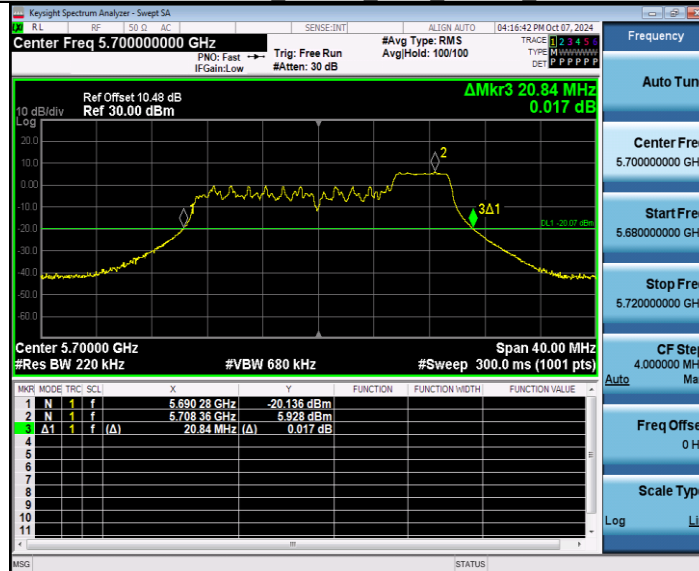
11AX20MIMO_Ant W0_5700_106Tone_RU54
