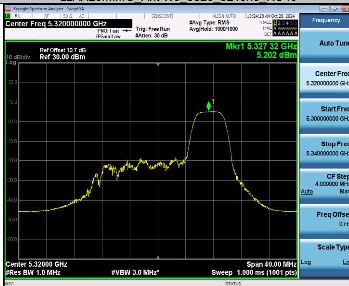
11AX20MIMO Ant W0 5320 106Tone RU54
