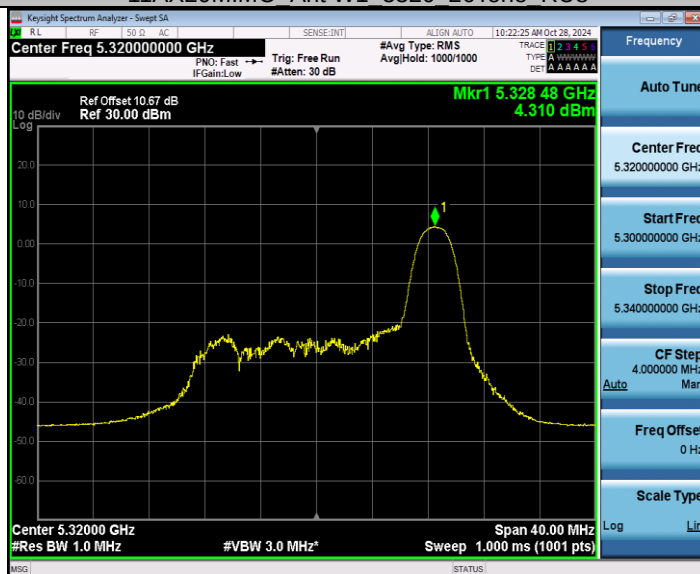
11AX20MIMO Ant W1 5320 52Tone RU40
