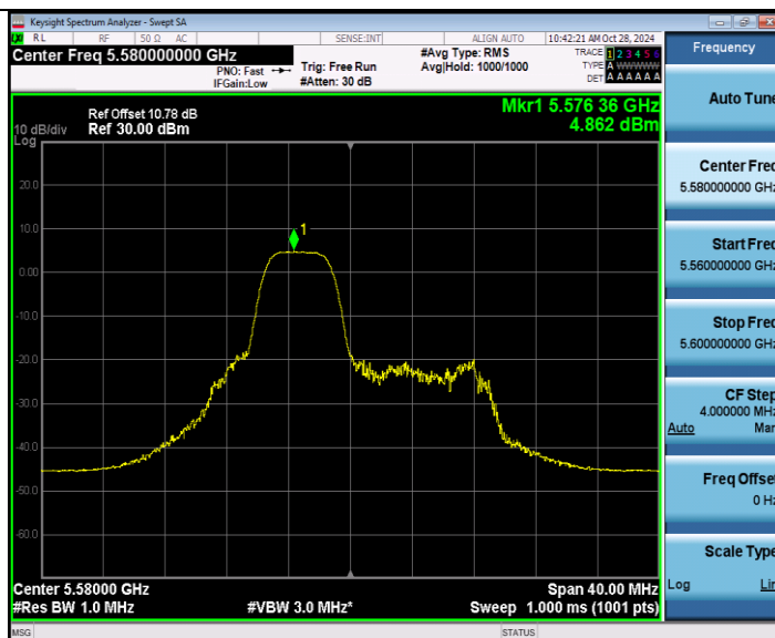
11AX20MIMO Ant W1 5580 106Tone RU53
