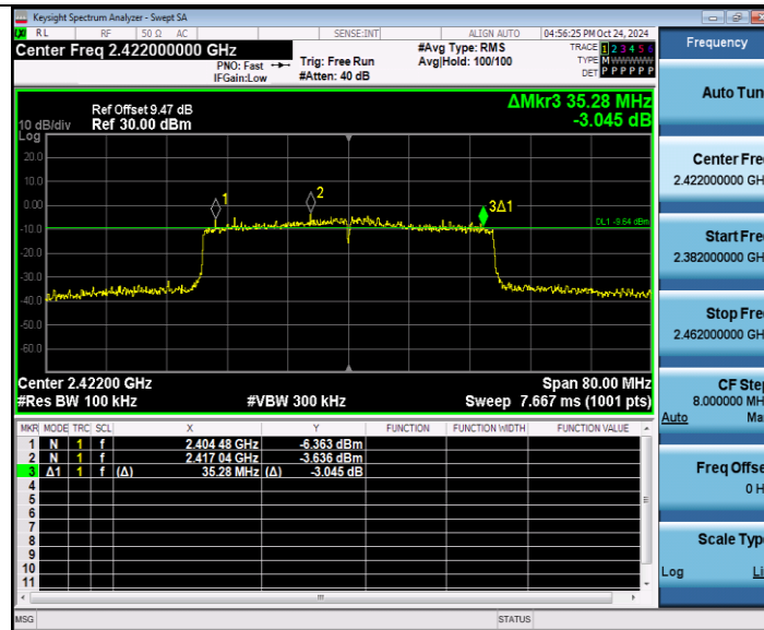
11AX40MIMO_Ant W1_2422
