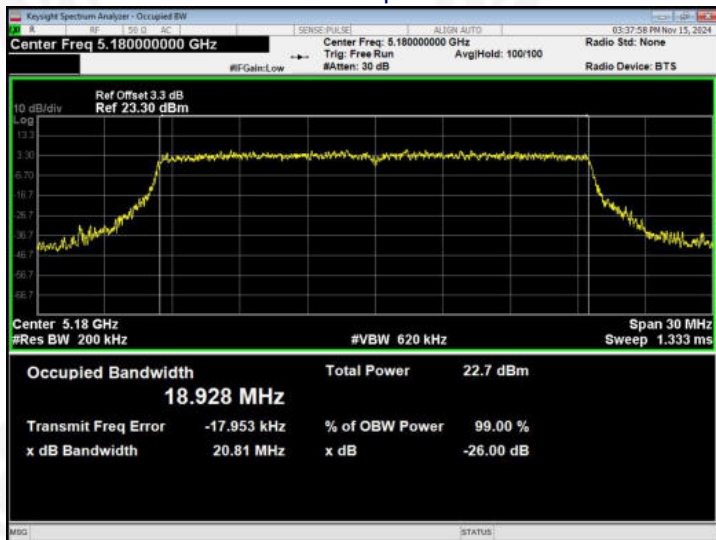
SISO ANT B - 802.11ac20
