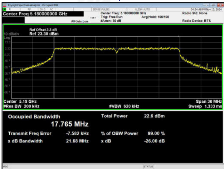
SISO ANT A - 802.11ac20
