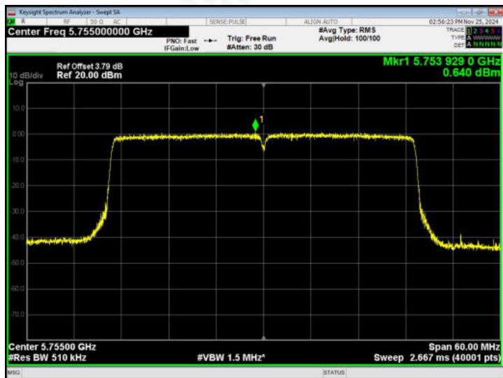
SISO ANT A - 802.11ax40 CH 151
