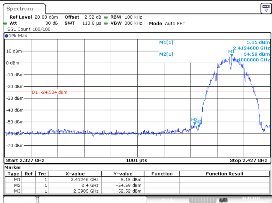
Band Edge NVNT b 2412MHz Ant2 Ref
