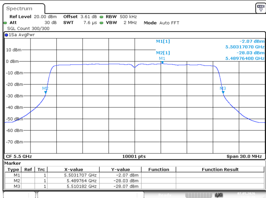
-26dB Bandwidth NVNT ax20 5500MHz Ant1
