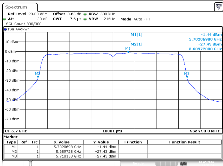
-26dB Bandwidth NVNT ax20 5700MHz Ant1
