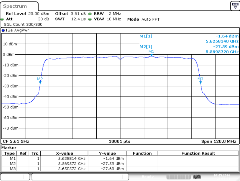
-26dB Bandwidth NVNT ac80 5610MHz Ant1
