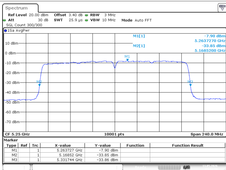
-26dB Bandwidth NVNT ac160 5250MHz Ant1
