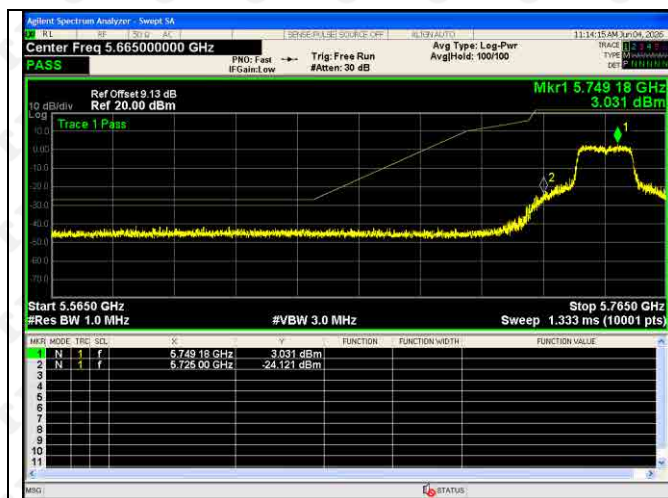
802.11(n40)-5755
