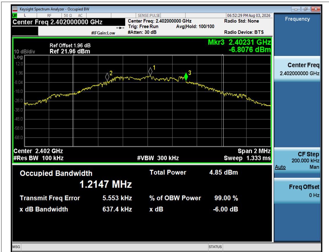
-6dB Bandwidth NVNT BLE 1M 2402MHz Ant1
