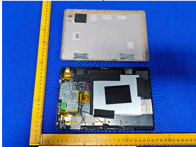
WWAN DIV Antenna
