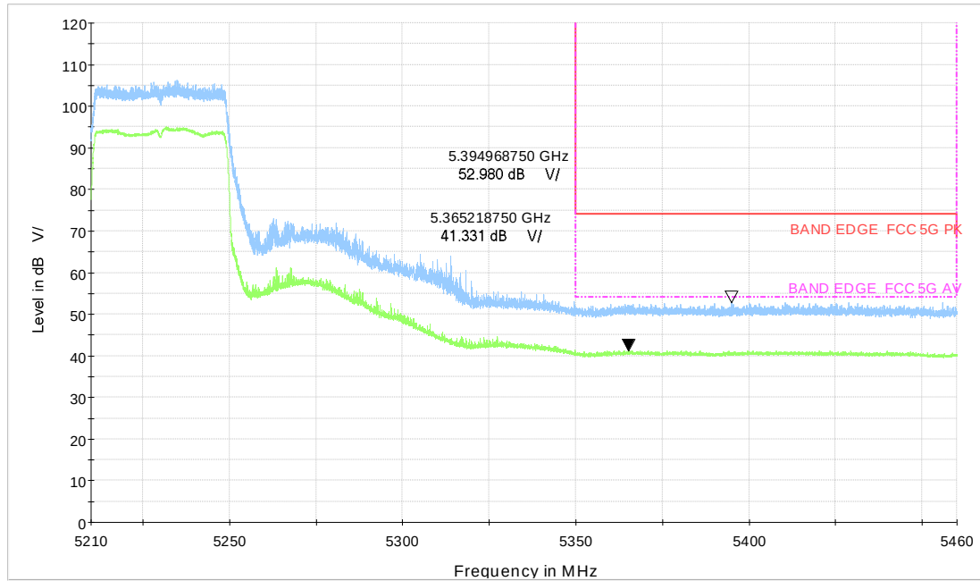
Wi-Fi 5GHz_BE40 CH46
