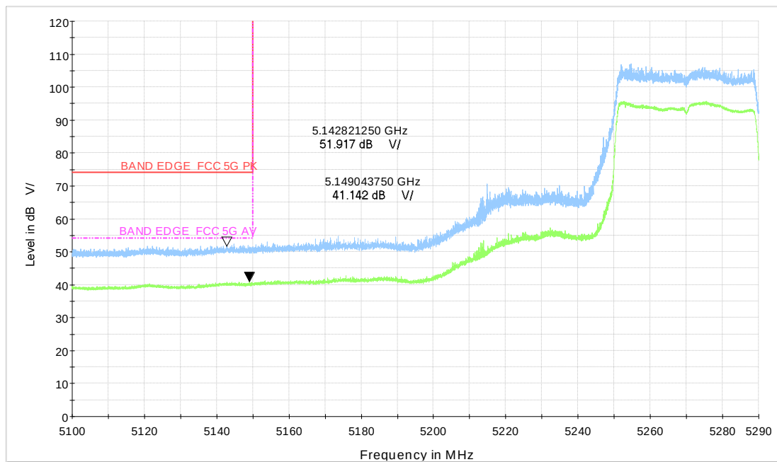
Wi-Fi 5GHz_BE40 CH54
