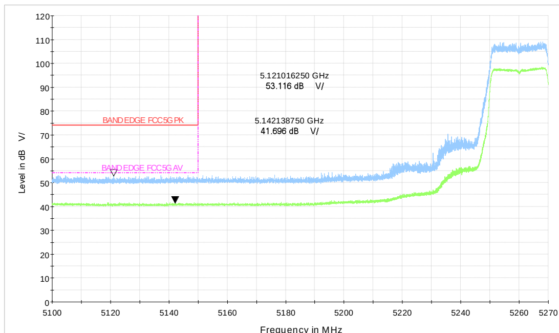
Wi-Fi 5GHz_ax20 CH52
