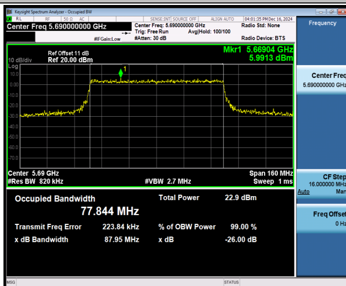
11AX80SISO_Ant1_5690
