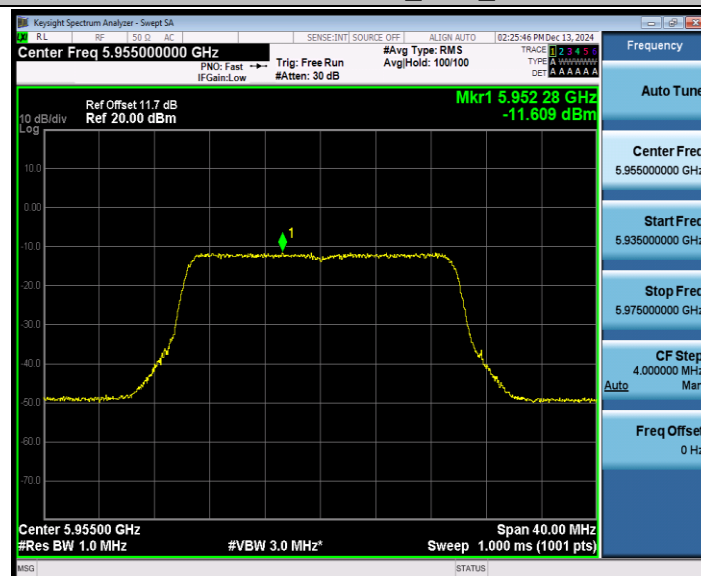
802.11be 20 MIMO_Ant2_5955
