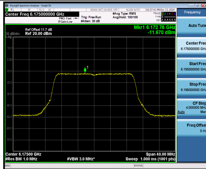
802.11be 20 MIMO_Ant2_6175
