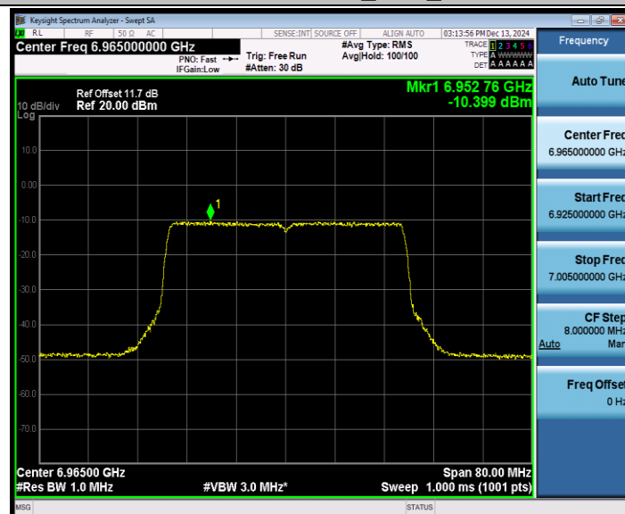
802.11be 40 MIMO_Ant2_6965
