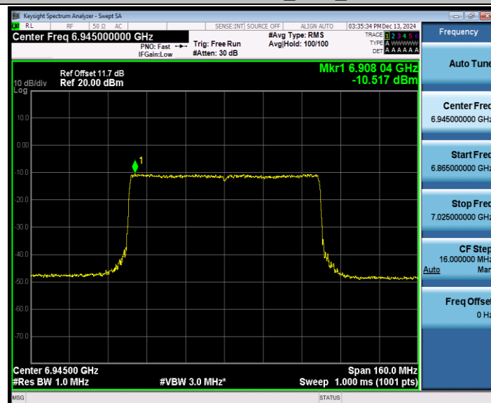
802.11be 80 MIMO_Ant2_6945
