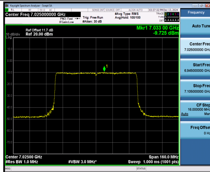
802.11be 80 MIMO_Ant2_7025
