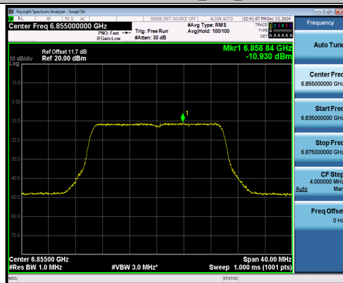
802.11be 20 MIMO_Ant2_6855
