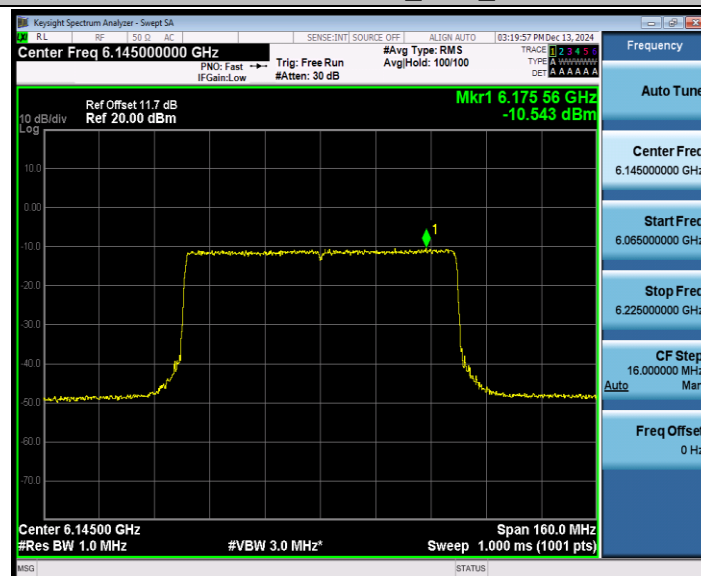
802.11be 80 MIMO_Ant2_6145
