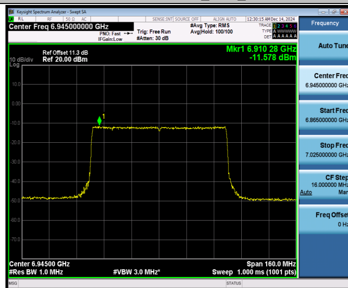
802.11be 80 MIMO_Ant1_7025
