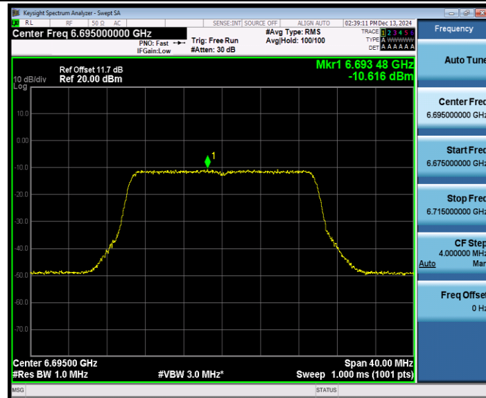
802.11be 20 MIMO_Ant2_6695
