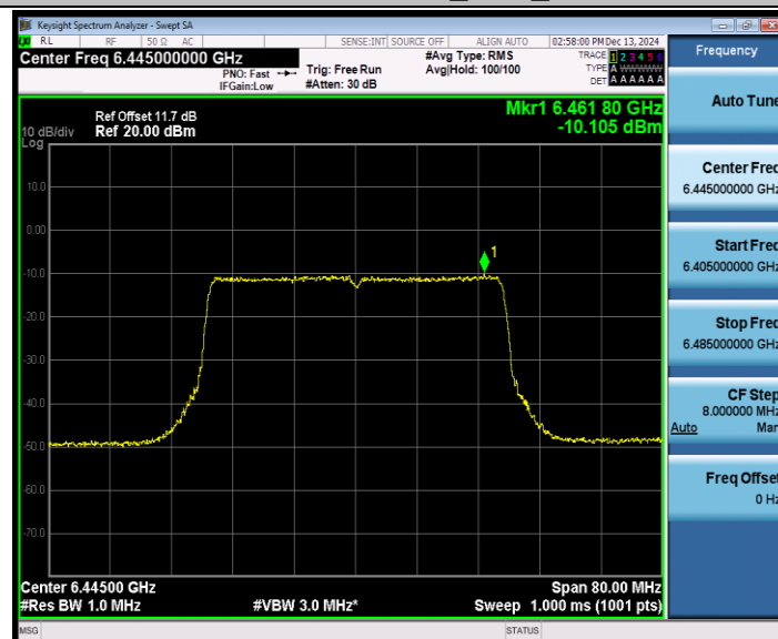
802.11be 40 MIMO_Ant2_6445
