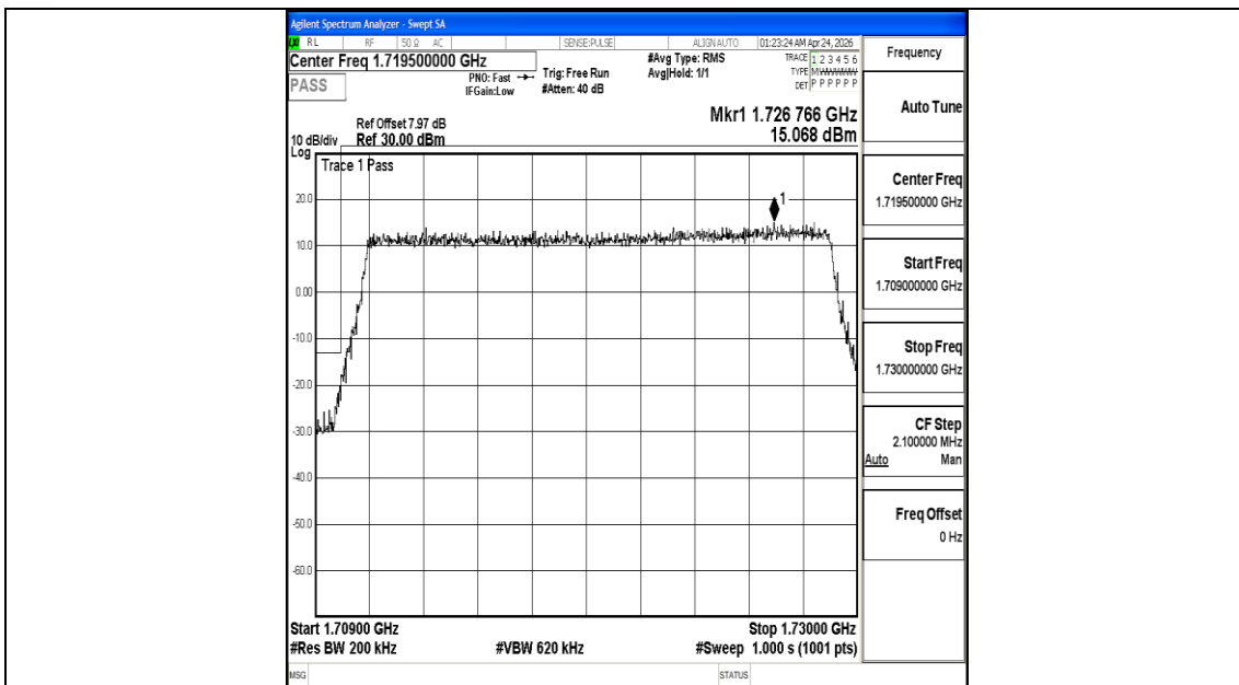
Band66_20MHz_QPSK_132072_100RB#0
