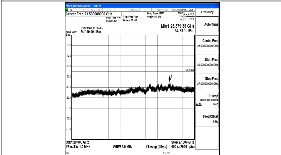
Band7_20MHz_QPSK_20850_1RB#0_20000~27000_20000~27000
