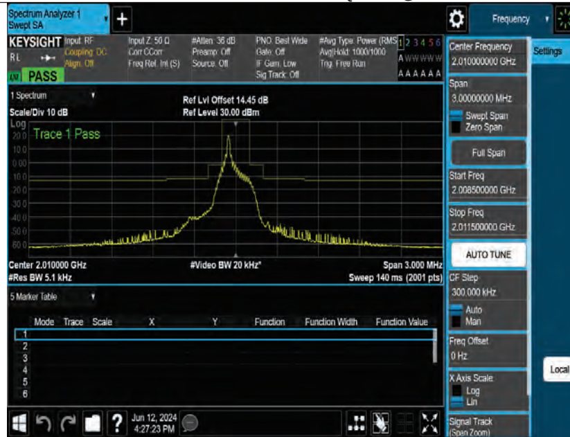
Band23-15kHz-MASK-M-QPSK-1@10
