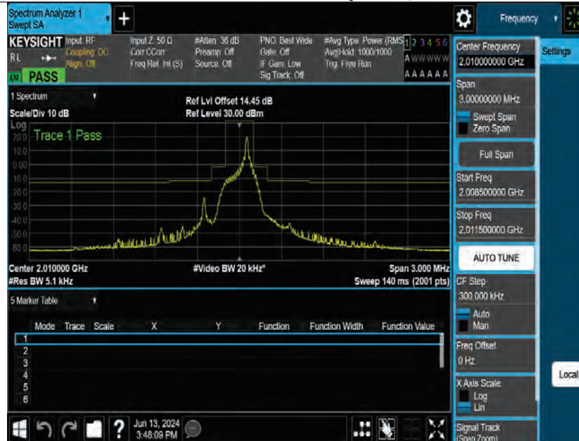
Band23-15kHz-MASK-M-QPSK-1@10
