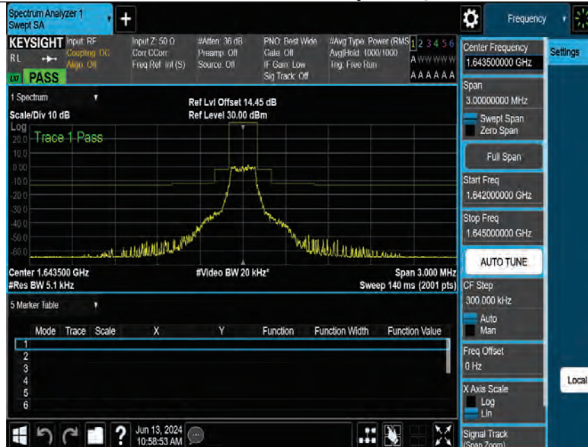
Band255-15kHz-MASK-M-QPSK-12@0
