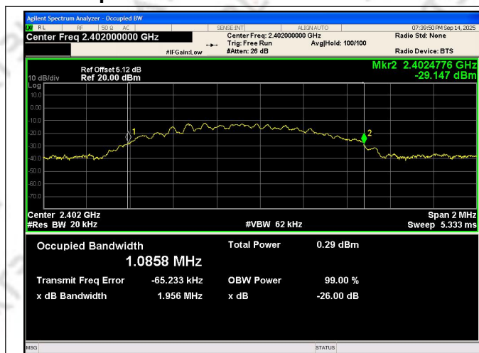
BLE 1M_Channel 0
