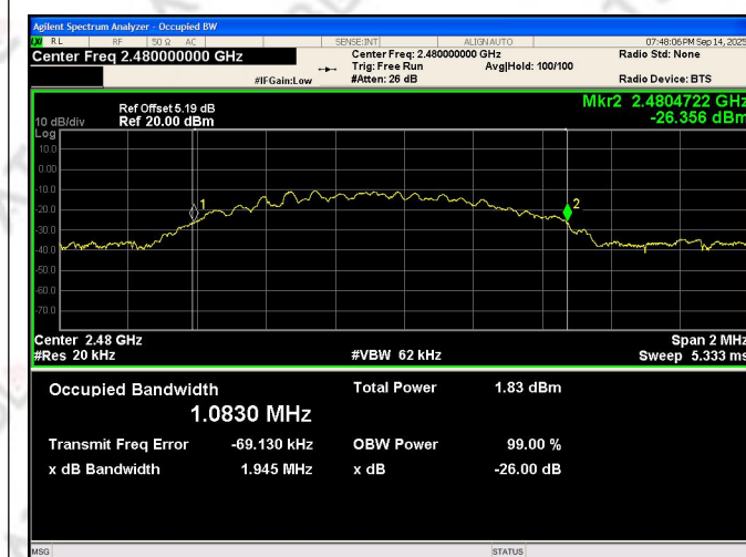
BLE 1M_Channel 39
