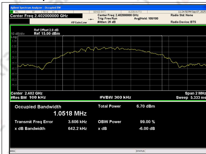
BLE 1M_Channel 0
