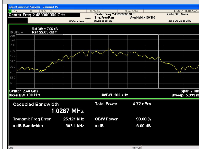
BLE 1M_Channel 39
