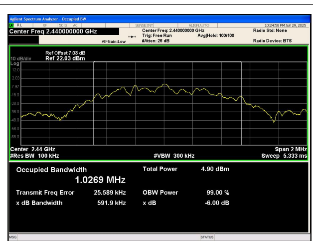
BLE 1M_Channel 19
