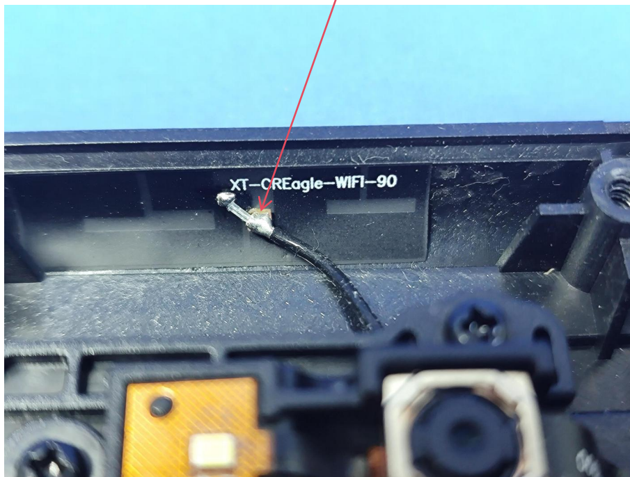
ANT 2(BT&2.4GWIFI&5GWIFI)
