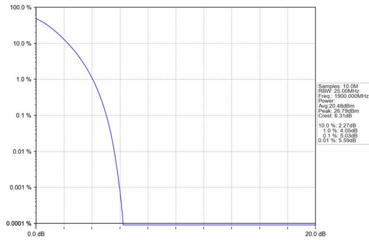
Band2_20MHz_QPSK_HCH_1900MHz_RB_100_0_NTNV
