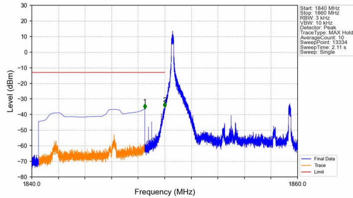
Band2_10MHz_QPSK_LCH_1855MHz_RB_1_0_NTNV
