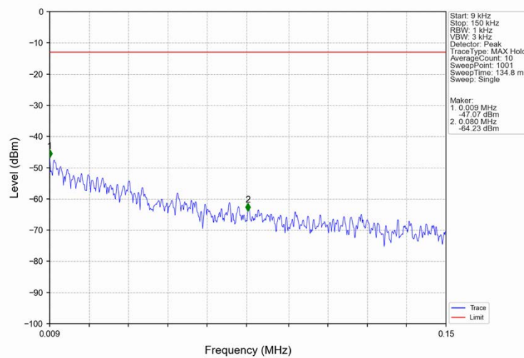
Band2_10MHz_QPSK_LCH_1855MHz_RB_1_0_NTNV
